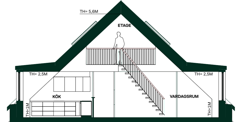
Sektion B, genom kök och vardagsrum
