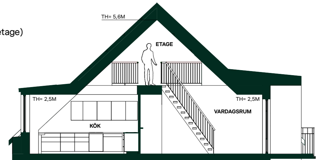
Sektion A, genom kök och vardagsrum
