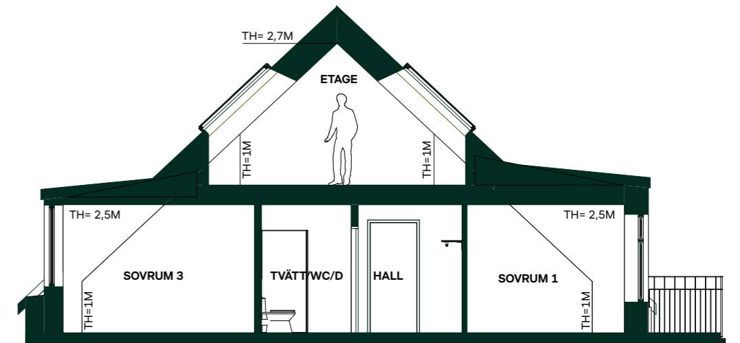
Sektion C genom sovrum
