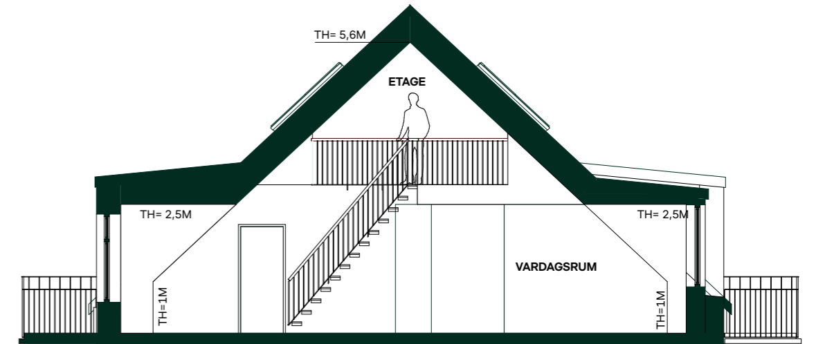
Sektion B genom vardagsrum
