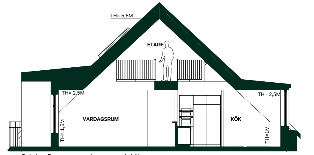
Sektion C, genom vardagsrum och kök
