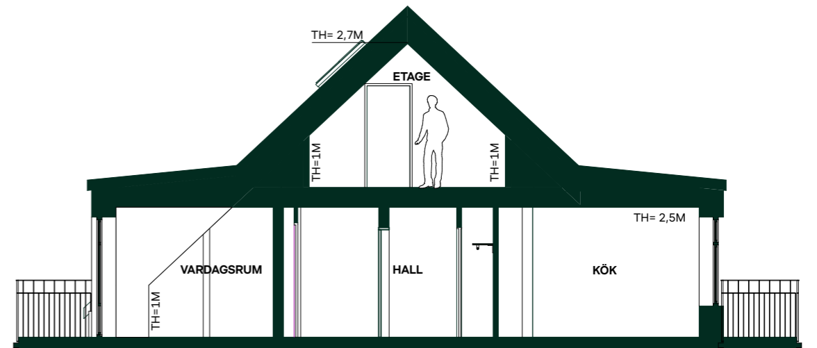
Sektion C, genom vardagsrum och kök
