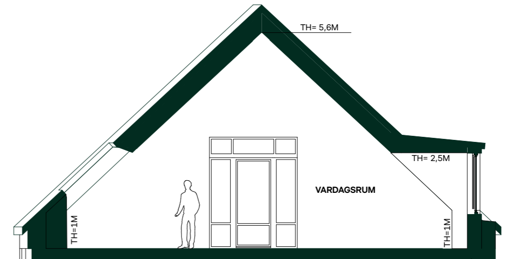
Sektion B, genom vardagsrum och kök
