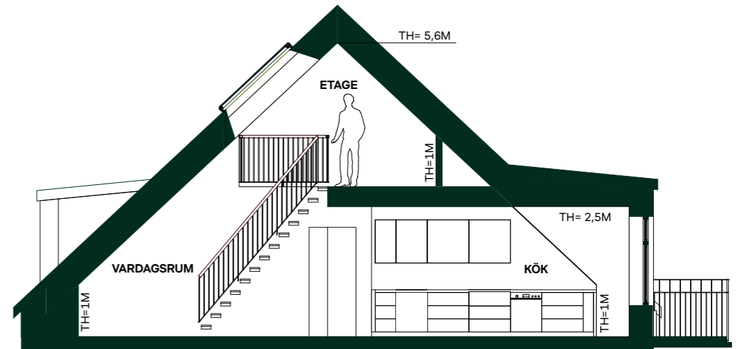
Sektion B, genom vardagsrum och kök
