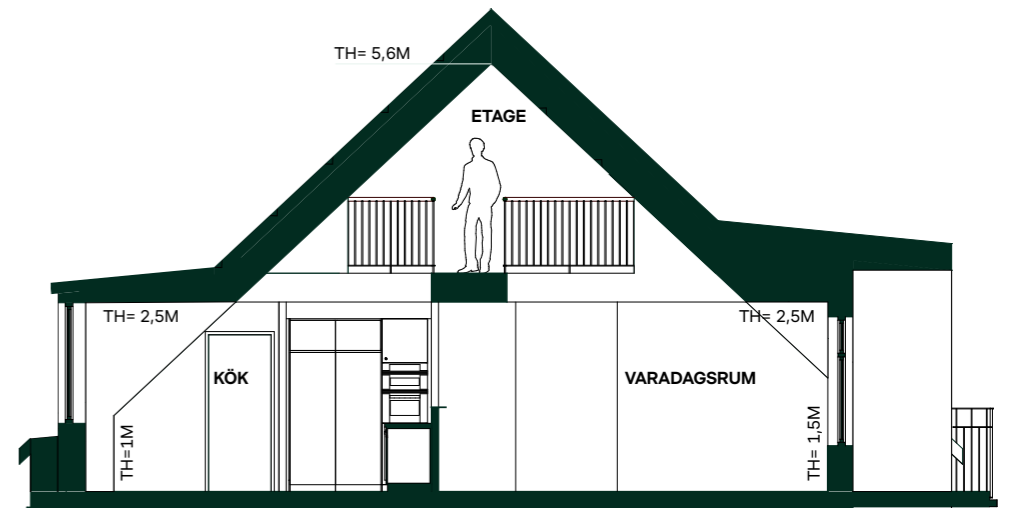
Sektion C, genom vardagsrum och kök
