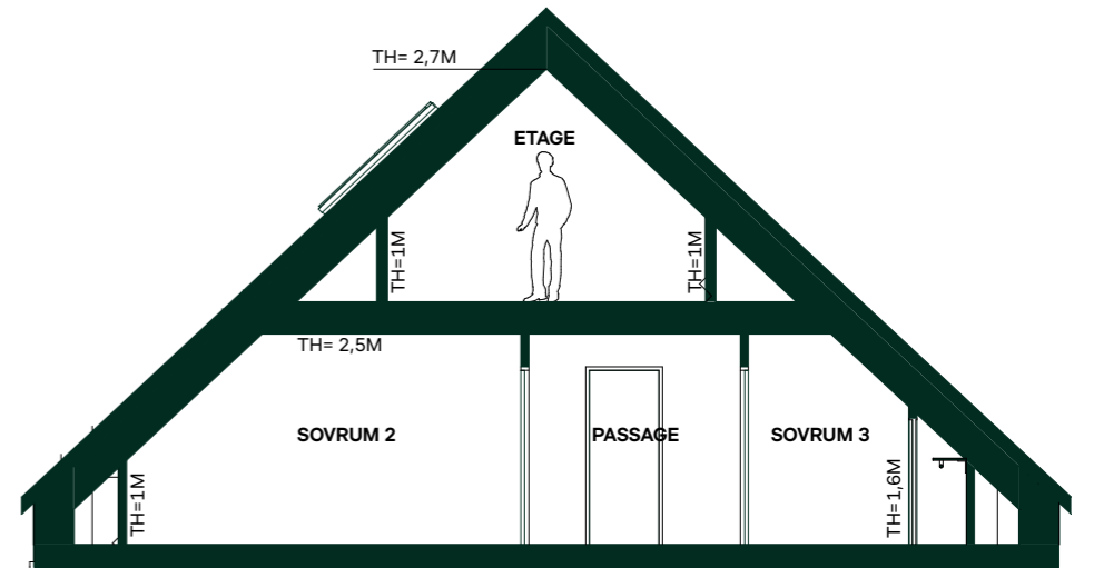
Sektion B, genom sovrums 2 och 3
