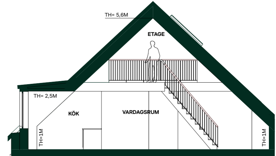
Sektion A, genom kök och vardagsrum
