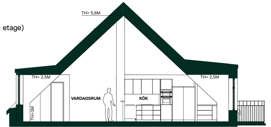
Sektion A genom vardagsrum och kök
