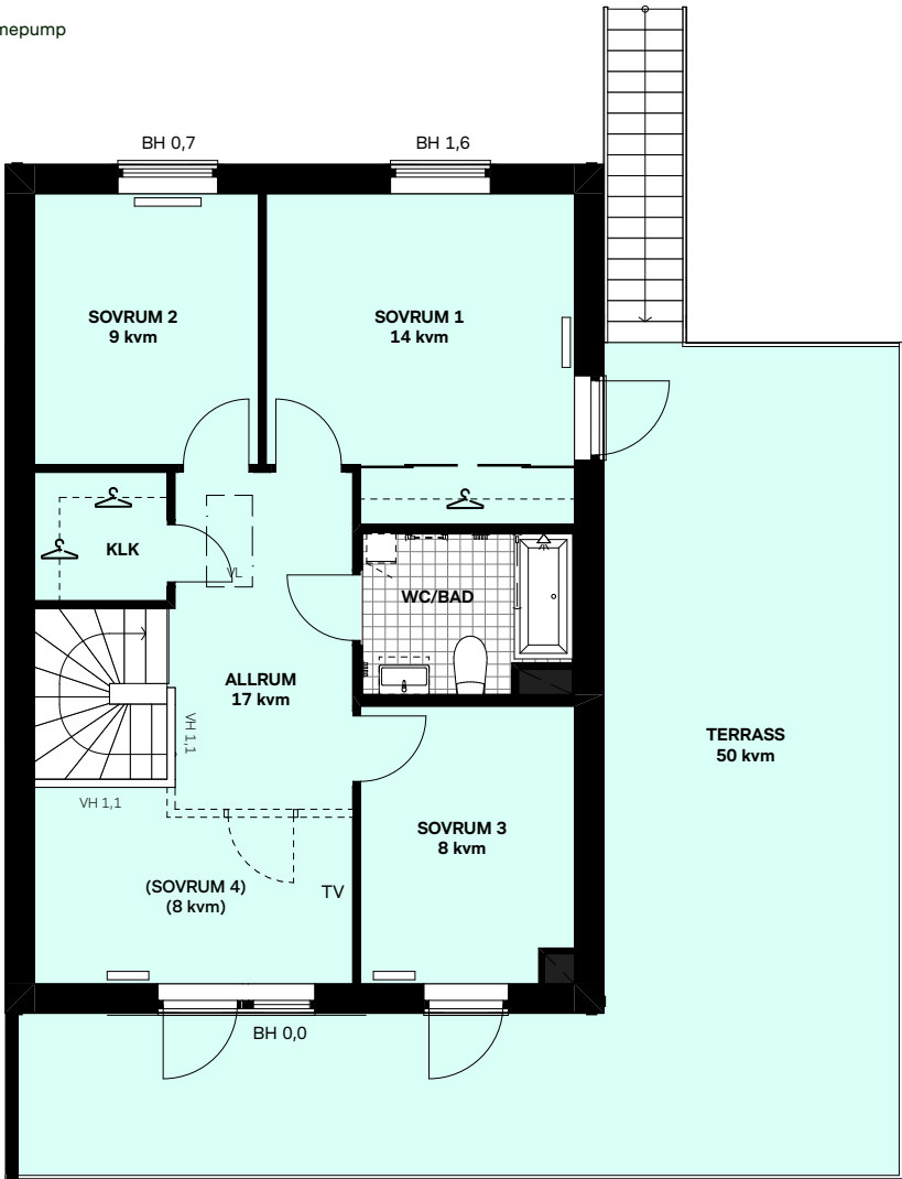
Övervåning
