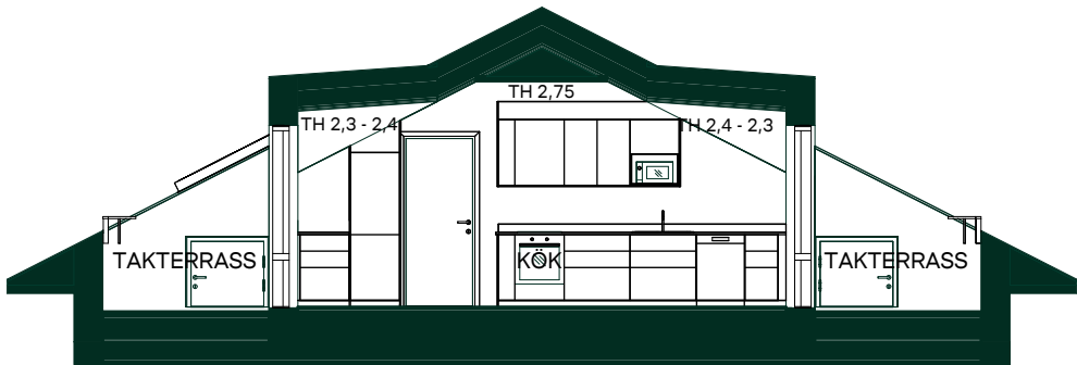
Sektion B-B
