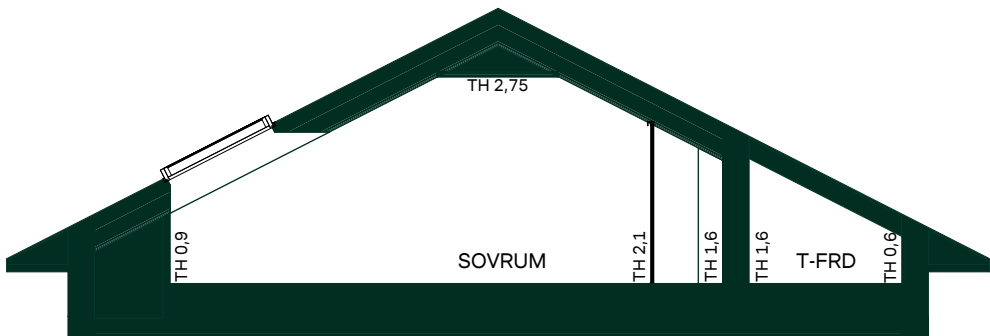
Sektion D-D
