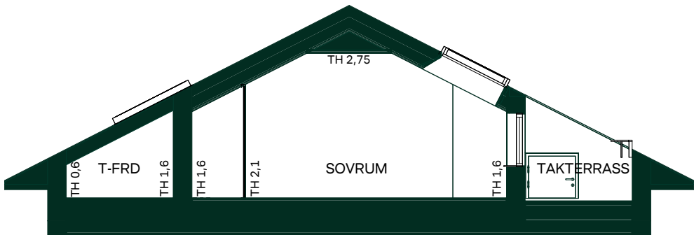
Sektion C-C
