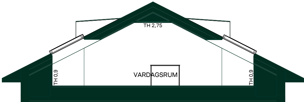
Sektion A-A
